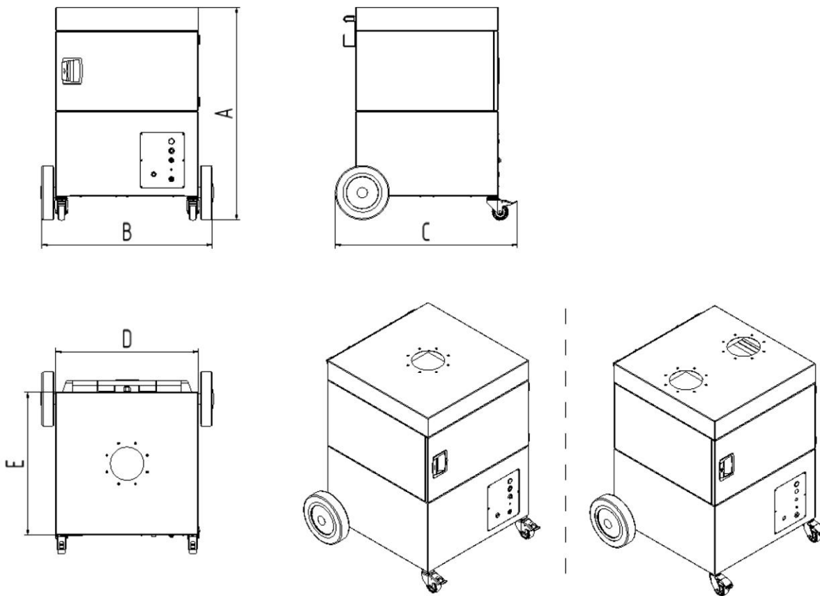
Fig. 9 : Fiches dimensionnelles 60650 + 60650DA
